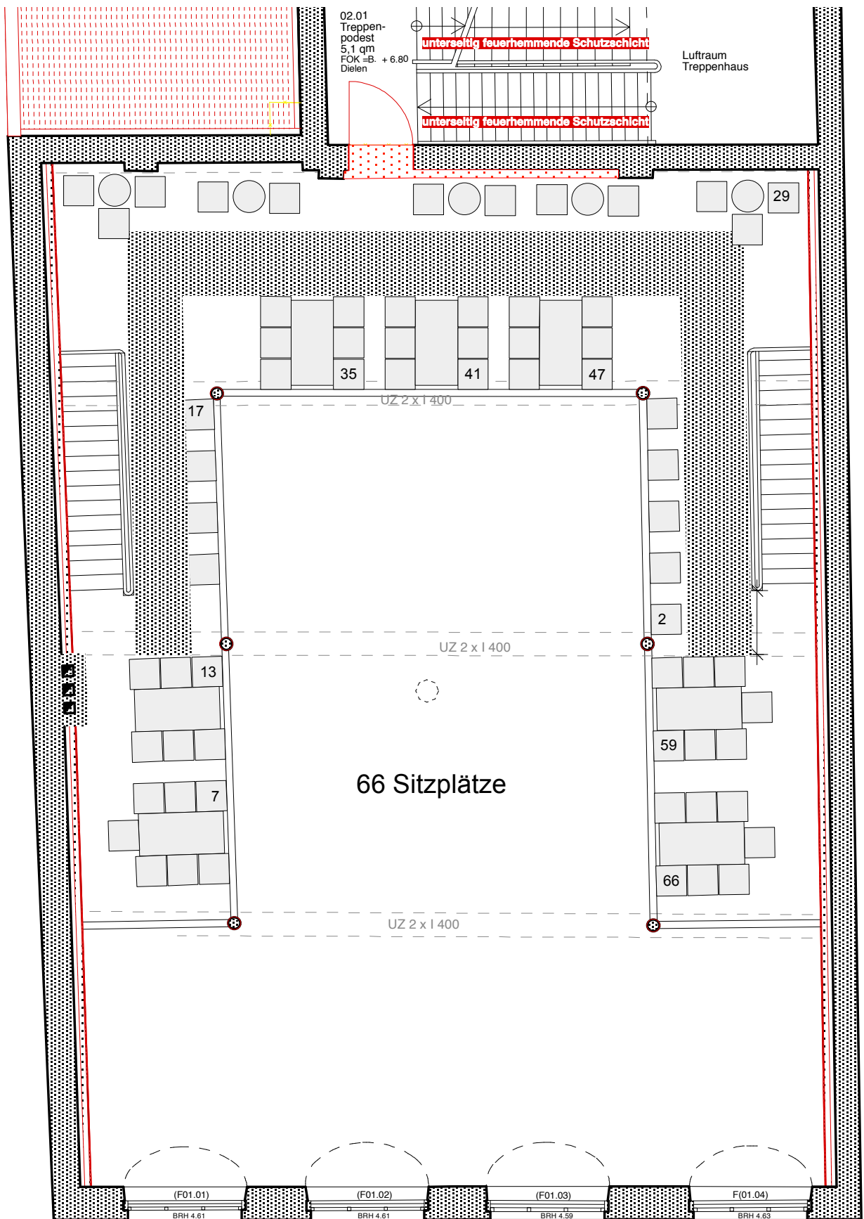
Galeriegeschoß - Bankettbestuhlung -
